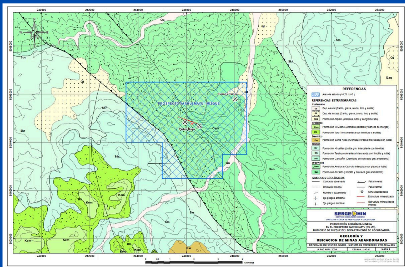
Mapa geológico base con delimitación del área del prospecto Yarhui Mayu. (línea azul)
