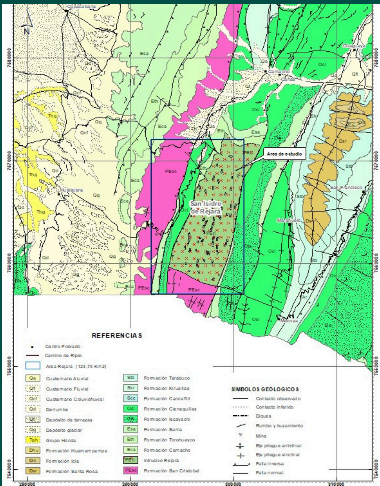
Mapa geológico del distrito de Rejara - Tarija
