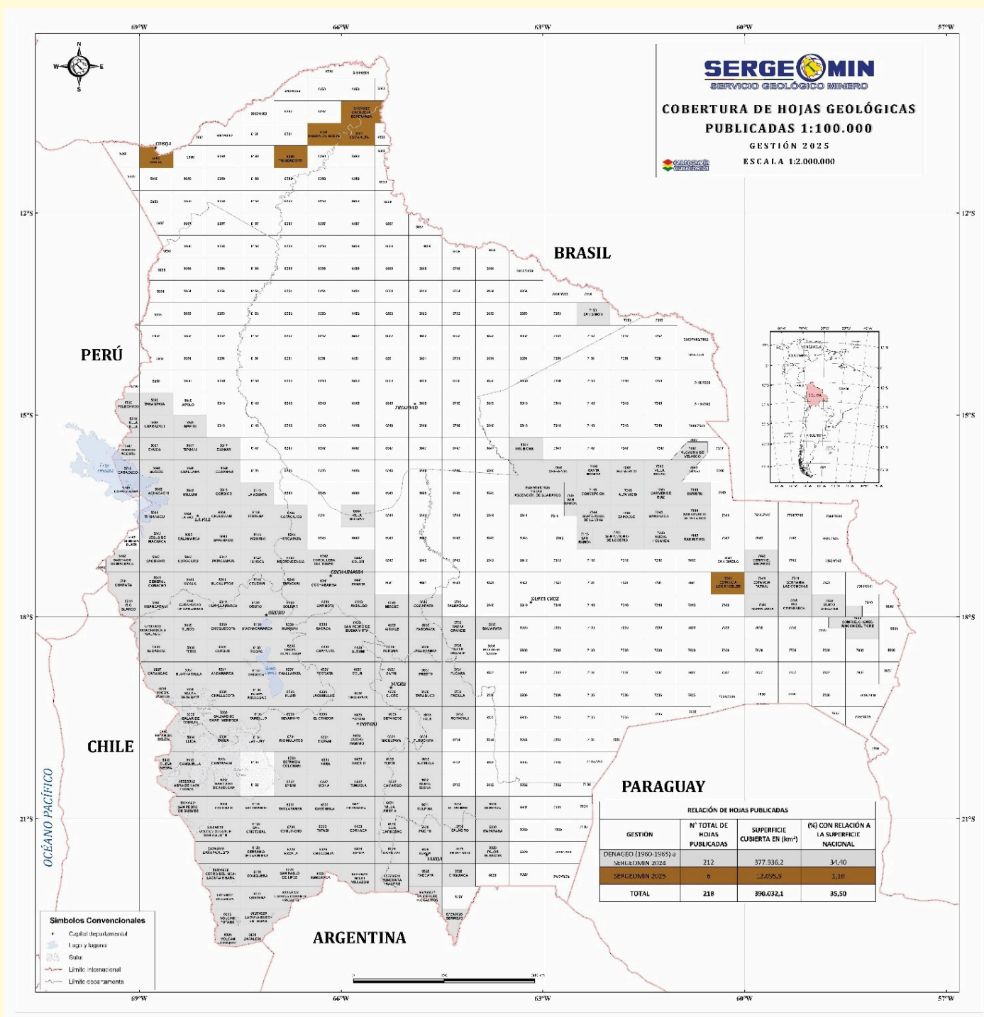
MAPA DE COBERTURA DE HOJAS GEOLOGICAS ESCALA 1:100.000.
