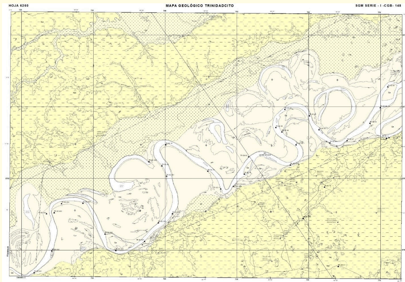
Mapa geológico hoja 6220 Trínadacito.
